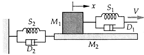
図1 摩擦振動モデル
